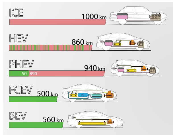
Reichweiten elektr mobiler Antriebskonzepte, Quelle: WWU/MEET
