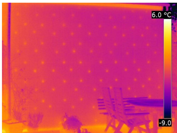
Dalmatiner-Effekt durch die Dübel beim Wärmedämmverbundsystem (WDVS)
