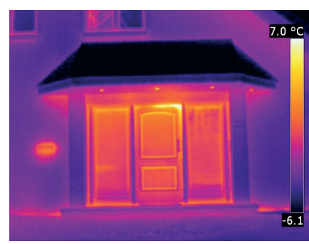
Nicht dicht schließende Haustür
