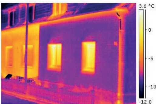
Thermografie eines gedämmten und nicht gedämmten Hauses. Allerdings wurde die Fensterlaibung nicht gedämmt.
